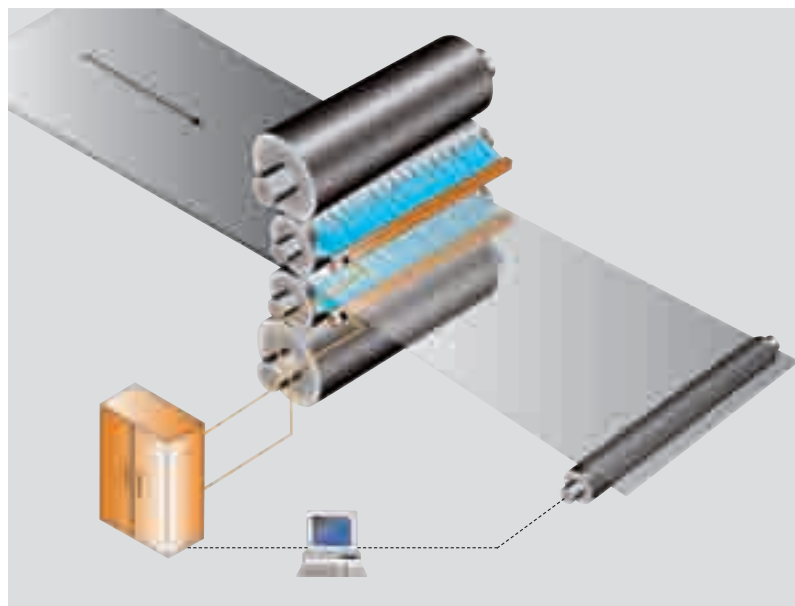
Elektrisch gesteuertes SELECTOSPRAY®-System mit EVA-Düsentechologie (25 mm/1", 50 mm/2")
